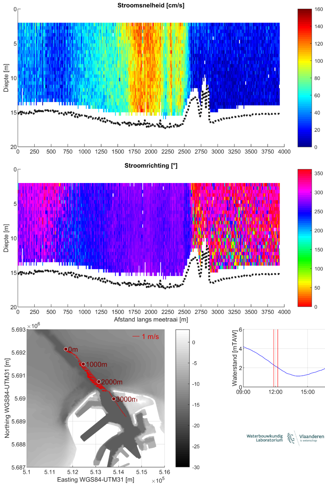
Figuur 15 – Stroomgegevens 09/08/2023 raai 10: snelheids grootte (top), -richting (midden) en diepte-gemiddelde vectoren (onder)
