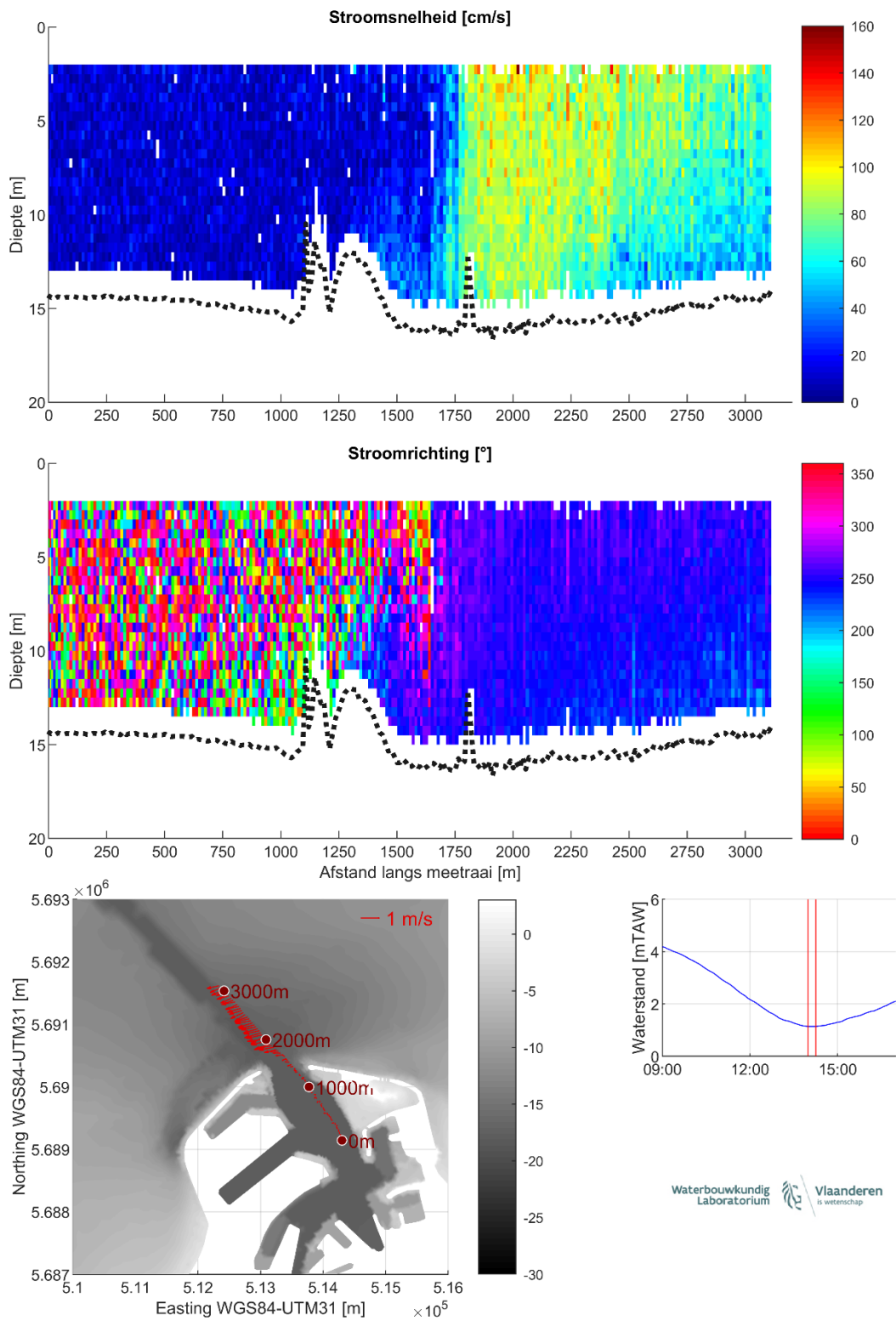
Figuur 22 – Stroomgegevens 09/08/2023 raai 17: snelheids grootte (top), -richting (midden) en diepte-gemiddelde vectoren (onder)
