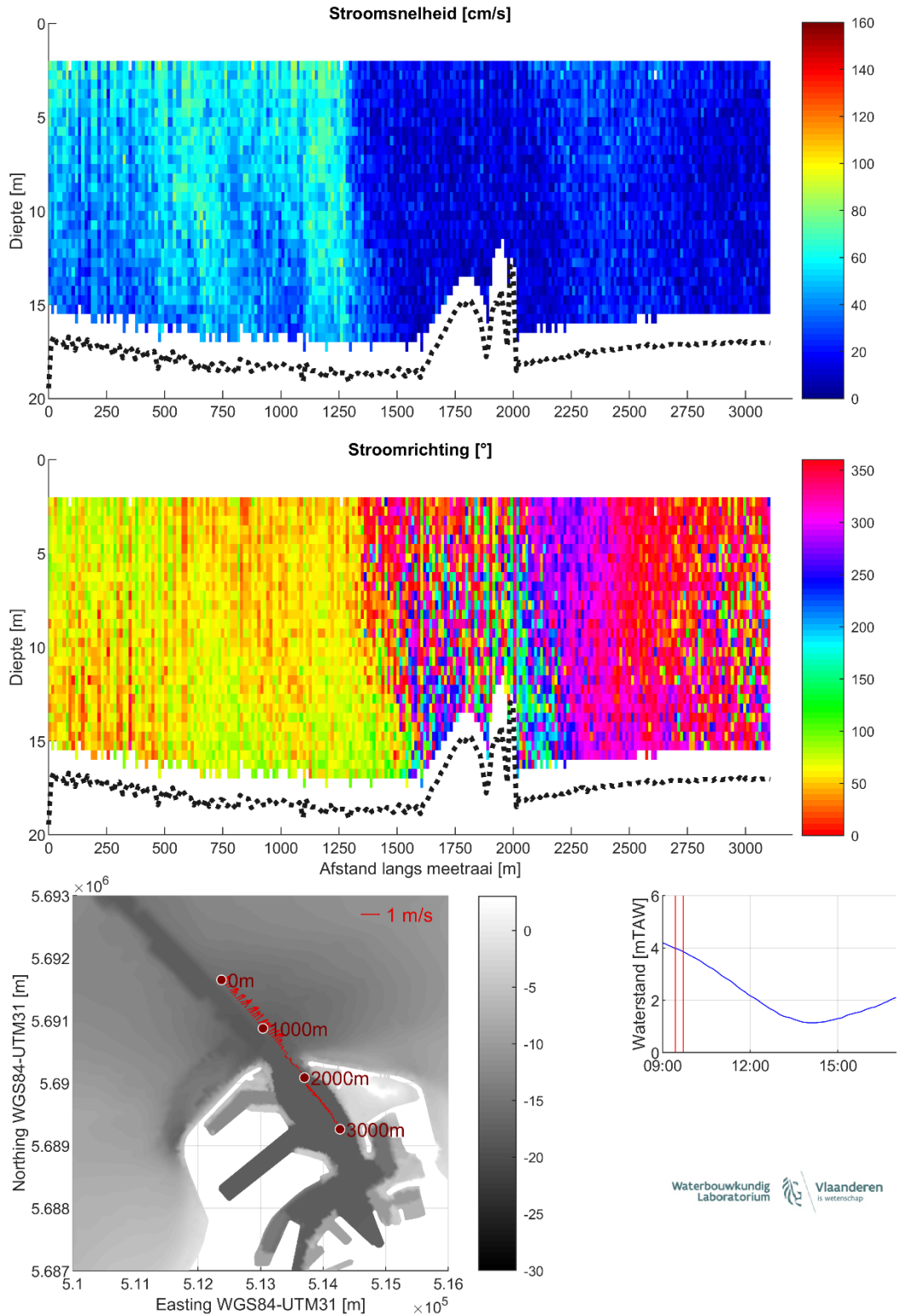
Figuur 7 – Stroomgegevens 09/08/2023 raai 2: snelheids grootte (top), -richting (midden) en diepte-gemiddelde vectoren (onder)
