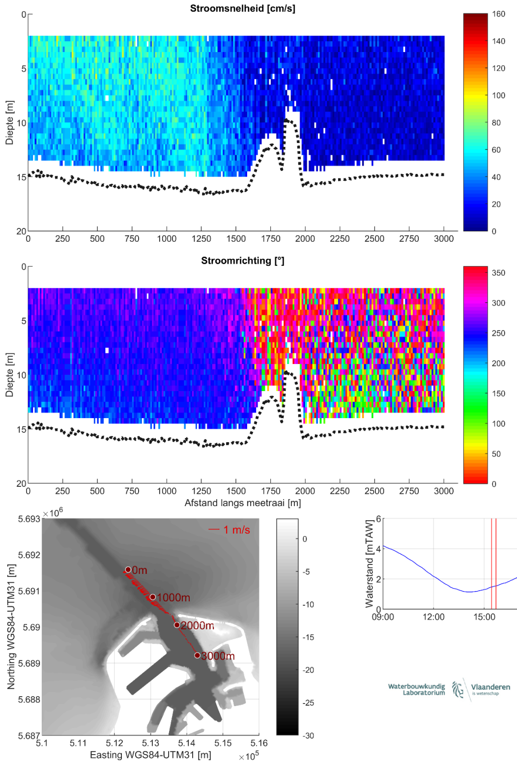
Figuur 27 – Stroomgegevens 09/08/2023 raai 22: snelheids grootte (top), -richting (midden) en diepte-gemiddelde vectoren (onder)
