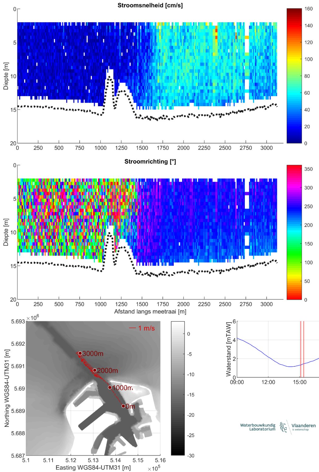
Figuur 26 – Stroomgegevens 09/08/2023 raai 21: snelheids grootte (top), -richting (midden) en diepte-gemiddelde vectoren (onder)
