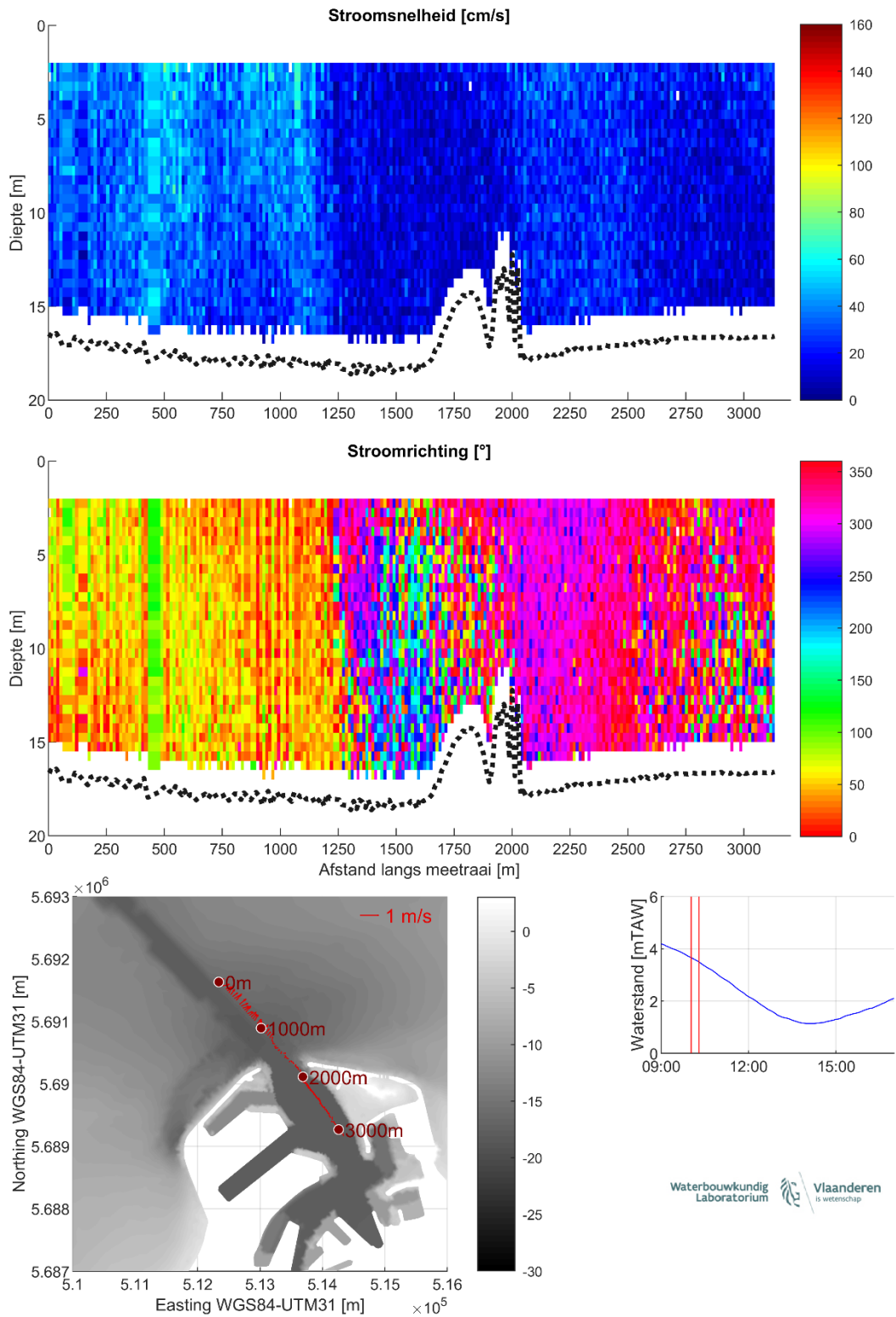
Figuur 9 – Stroomgegevens 09/08/2023 raai 4: snelheids grootte (top), -richting (midden) en diepte-gemiddelde vectoren (onder)
