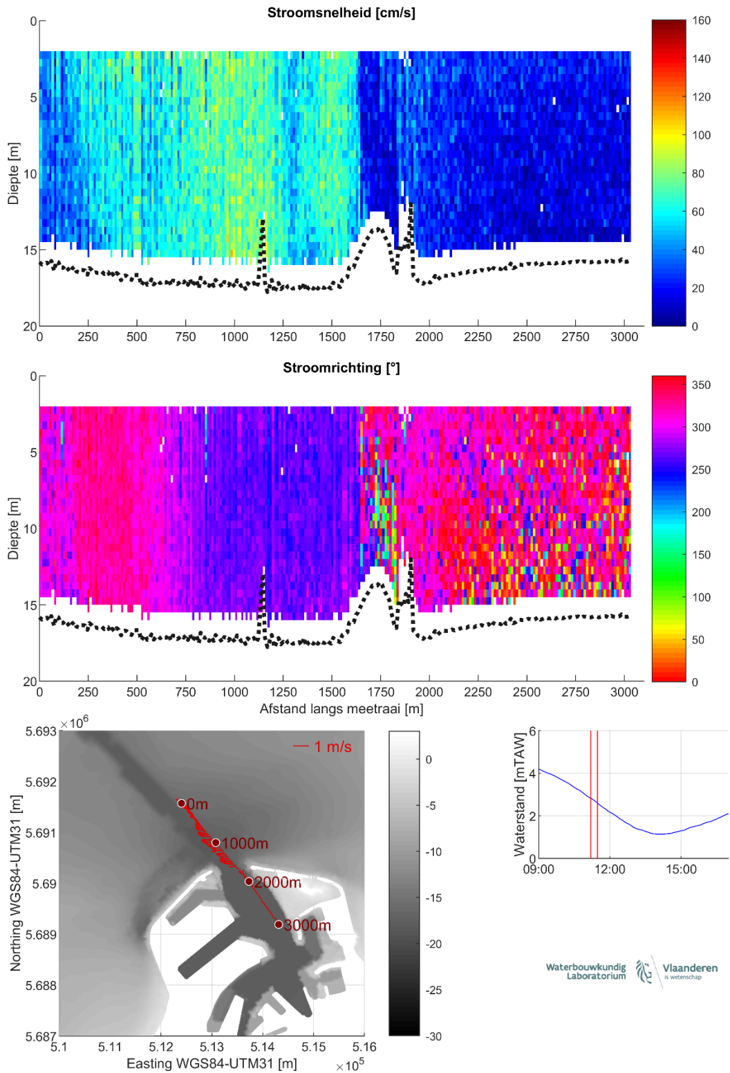
Figuur 13 – Stroomgegevens 09/08/2023 raai 8: snelheids grootte (top), -richting (midden) en diepte-gemiddelde vectoren (onder)
