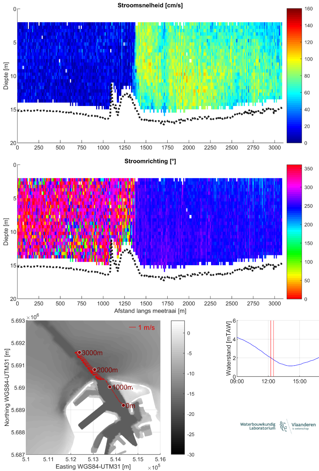
Figuur 16 – Stroomgegevens 09/08/2023 raai 11: snelheids grootte (top), -richting (midden) en diepte-gemiddelde vectoren (onder)
