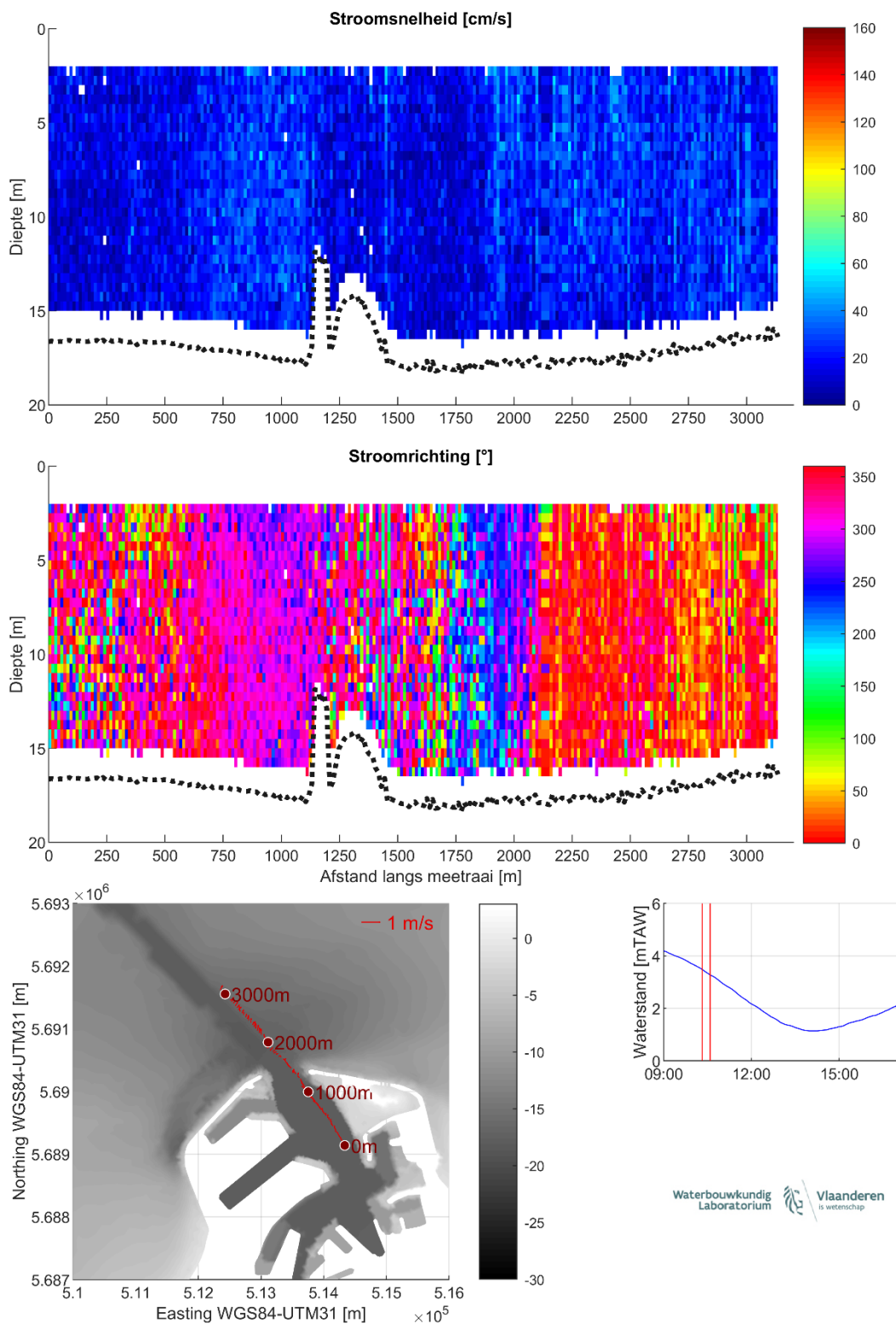
Figuur 10 – Stroomgegevens 09/08/2023 raai 5: snelheidsgrootte (top), -richting (midden) en diepte-gemiddelde vectoren (onder)
