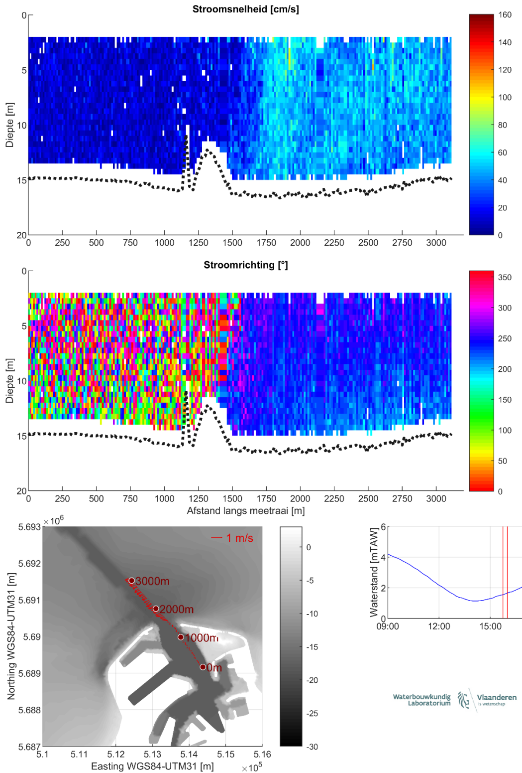
Figuur 28 – Stroomgegevens 09/08/2023 raai 23: snelheids grootte (top), -richting (midden) en diepte-gemiddelde vectoren (onder)
