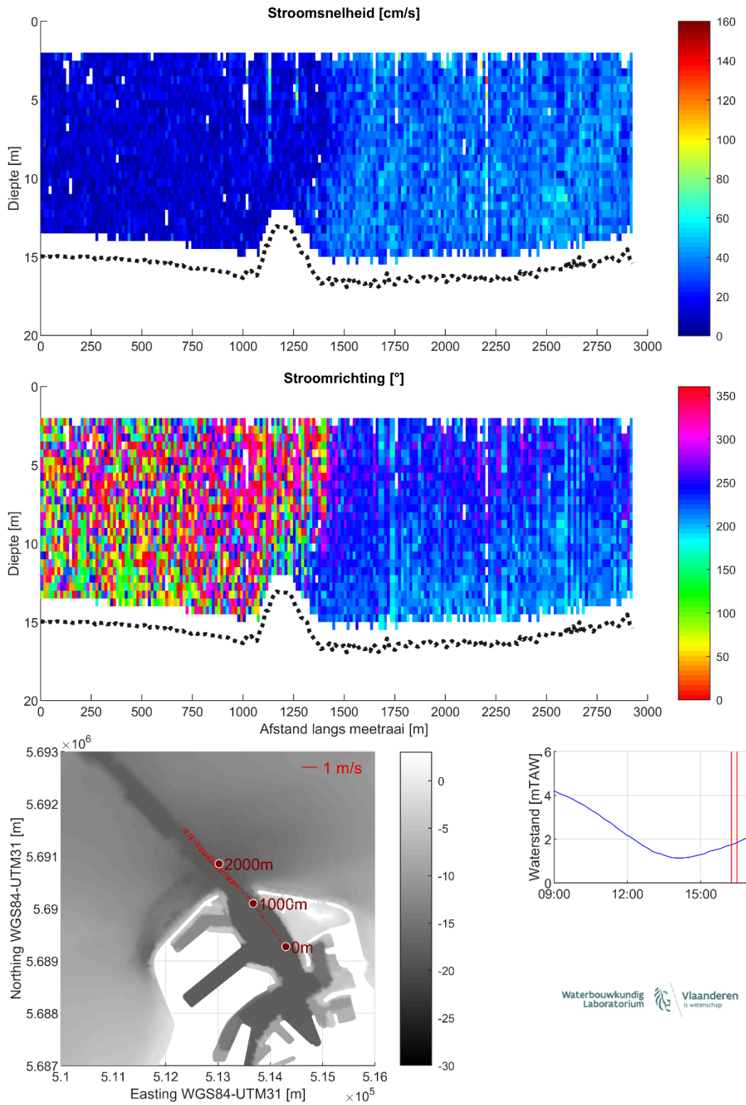
Figuur 30 – Stroomgegevens 09/08/2023 raai 25: snelheids grootte (top), -richting (midden) en diepte-gemiddelde vectoren (onder)
