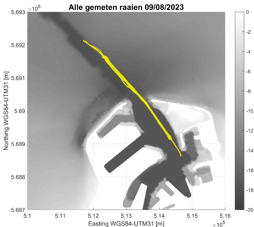
Figuur 3 – Ligging gemeten raaien op de meetdag 09/08/2023
