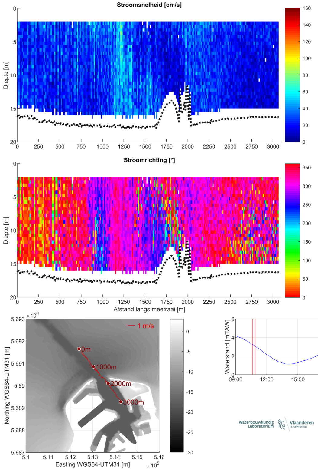
Figuur 11 – Stroomgegevens 09/08/2023 raai 6: snelheids grootte (top), -richting (midden) en diepte-gemiddelde vectoren (onder)
