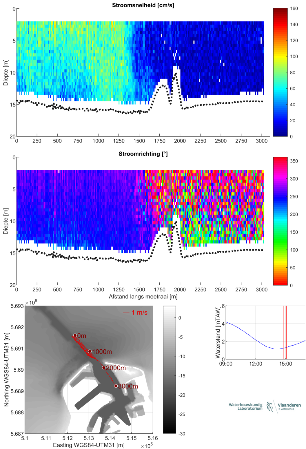
Figuur 25 – Stroomgegevens 09/08/2023 raai 20: snelheids grootte (top), -richting (midden) en diepte-gemiddelde vectoren (onder)
