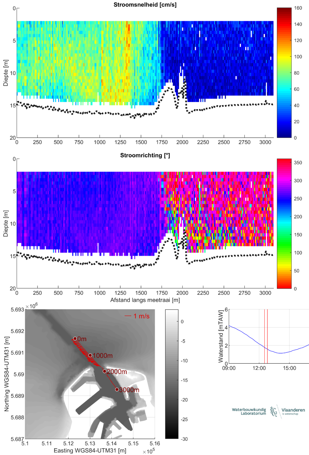
Figuur 17 – Stroomgegevens 09/08/2023 raai 12: snelheids grootte (top), -richting (midden) en diepte-gemiddelde vectoren (onder)
