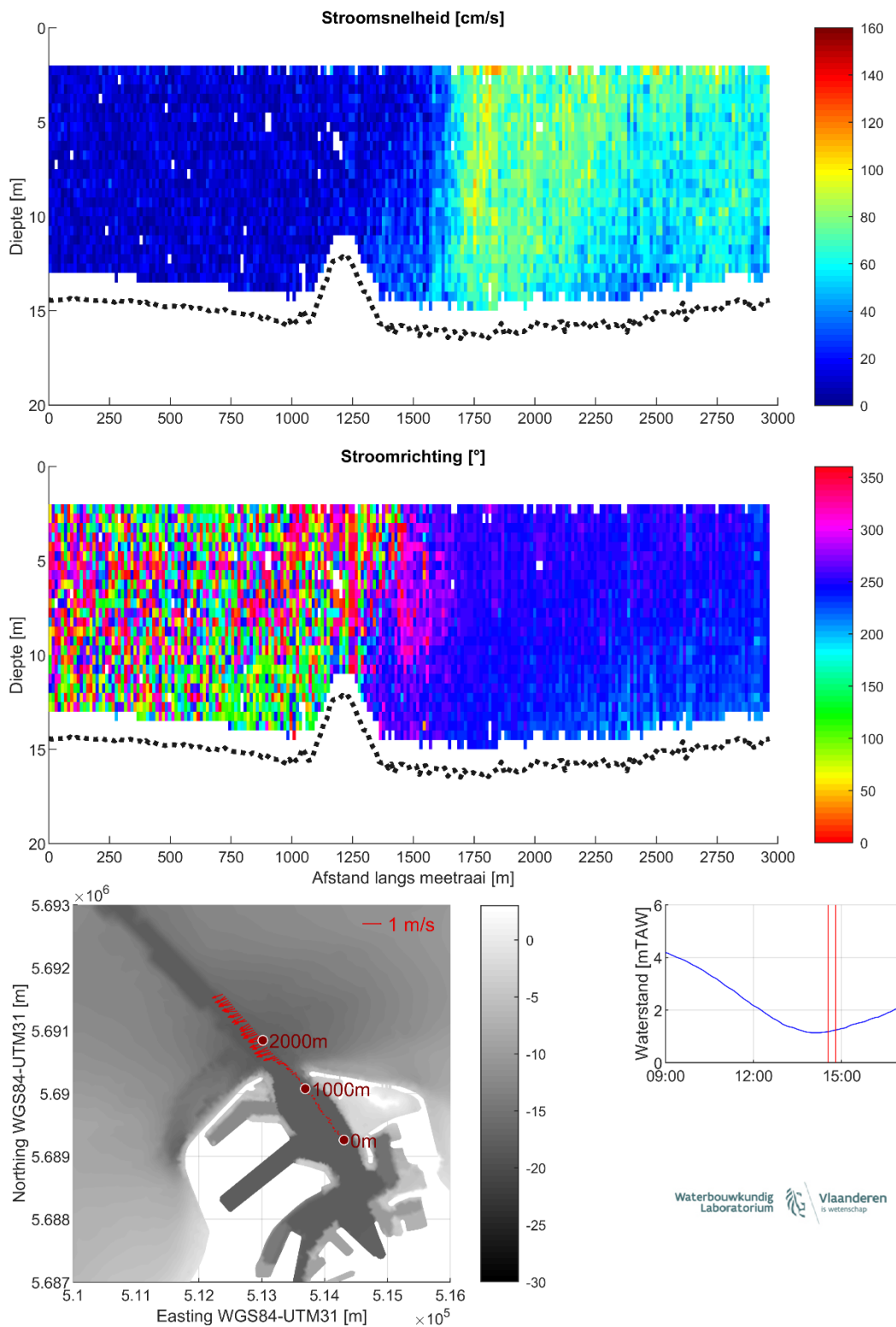
Figuur 24 – Stroomgegevens 09/08/2023 raai 19: snelheids grootte (top), -richting (midden) en diepte-gemiddelde vectoren (onder)
