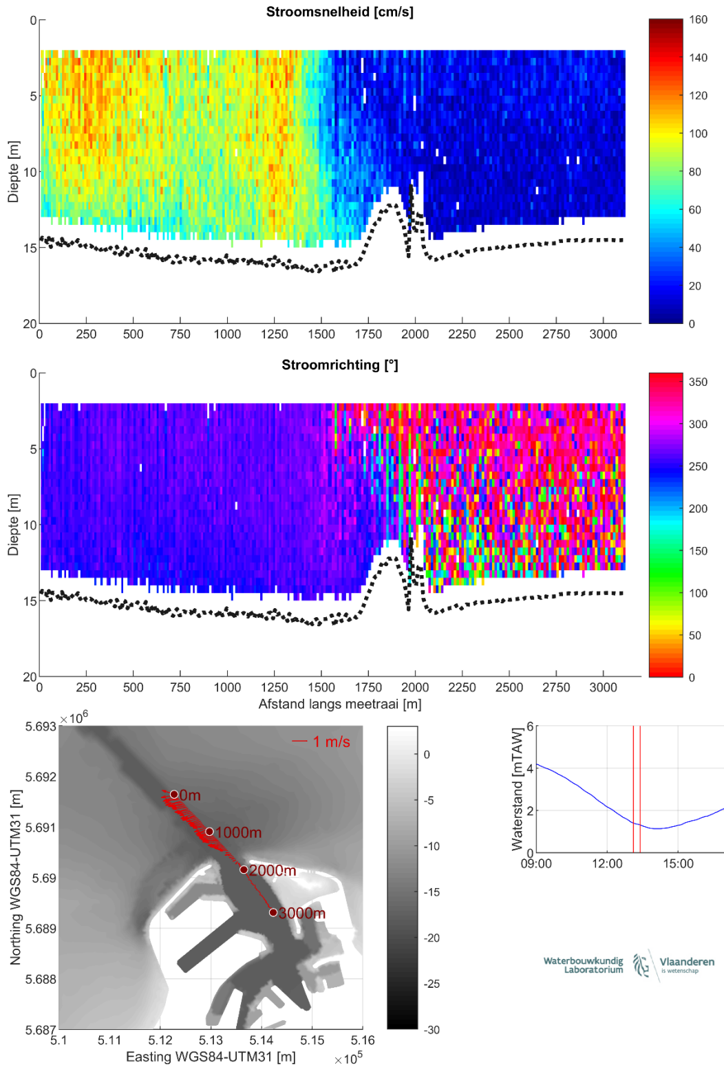
Figuur 19 – Stroomgegevens 09/08/2023 raai 14: snelheidsgrootte (top), -richting (midden) en diepte-gemiddelde vectoren (onder)
