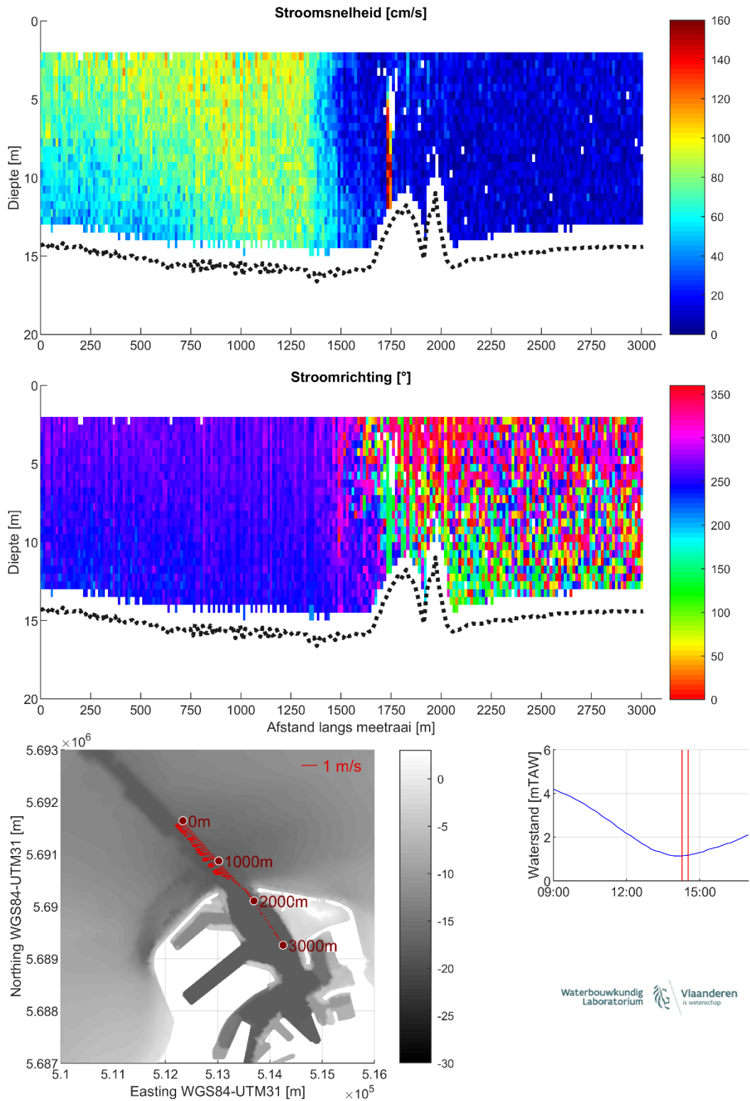
Figuur 23 – Stroomgegevens 09/08/2023 raai 18: snelheids grootte (top), -richting (midden) en diepte-gemiddelde vectoren (onder)
