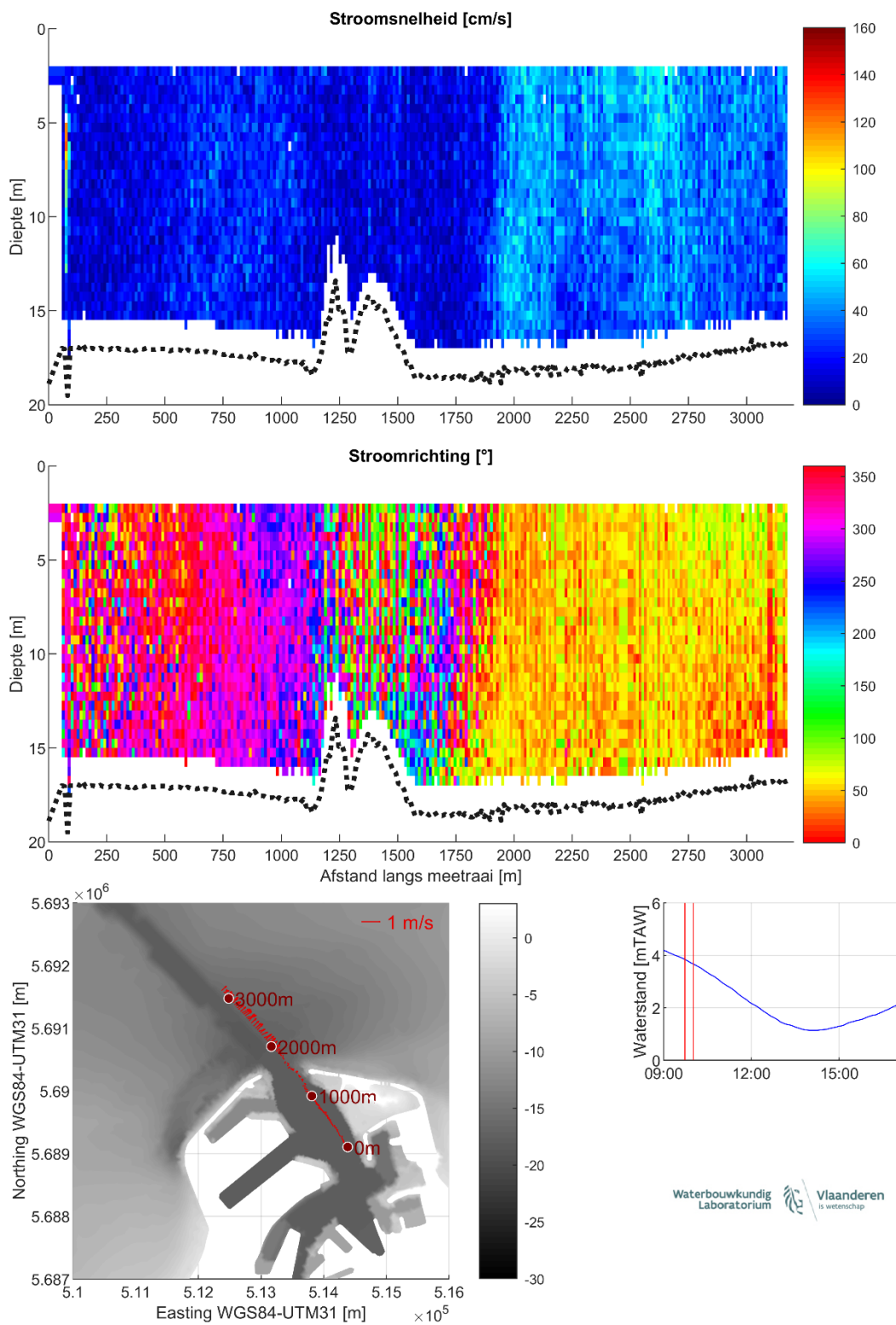
Figuur 8 – Stroomgegevens 09/08/2023 raai 3: snelheidsgroutte (top), -richting (midden) en diepte-gemiddelde vectoren (onder)
