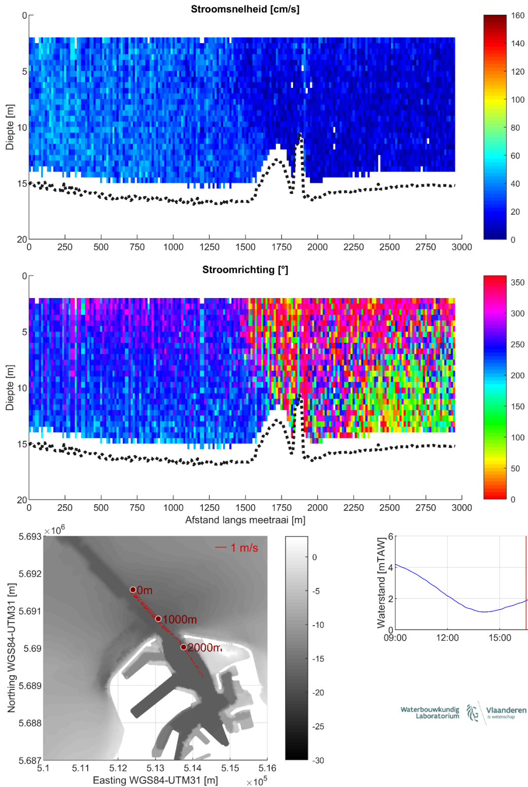
Figuur 31 – Stroomgegevens 09/08/2023 raai 26: snelheids grootte (top), -richting (midden) en diepte-gemiddelde vectoren (onder)
