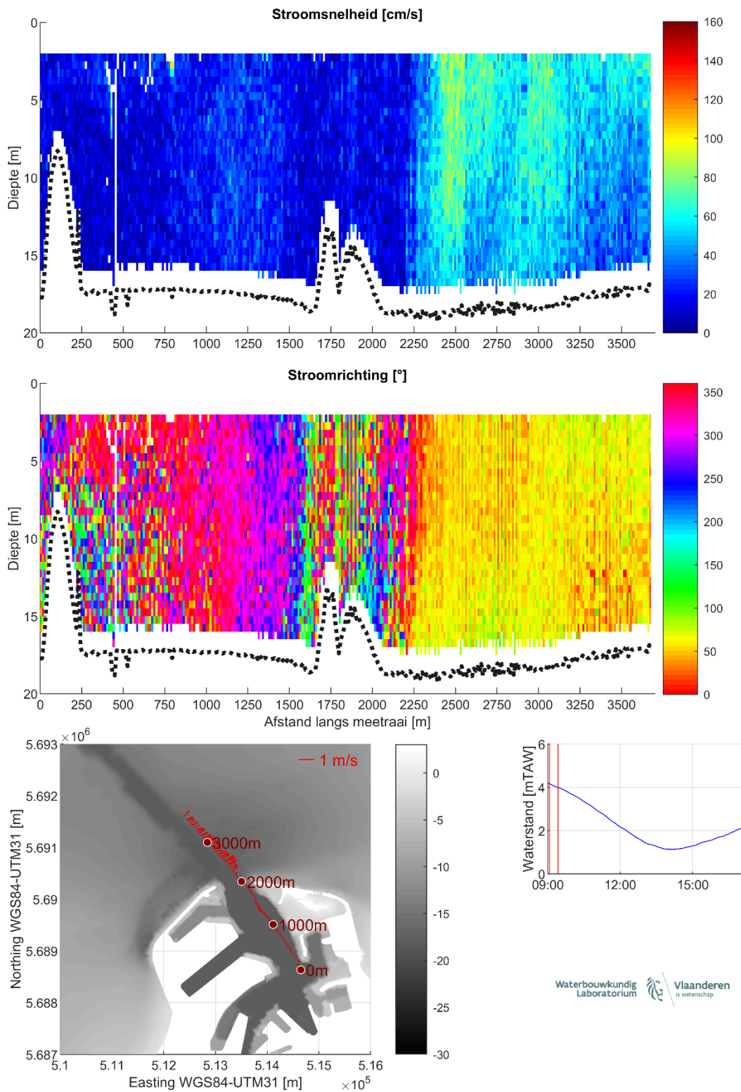
Figuur 6 – Stroomgegevens 09/08/2023 raai 1: snelheids grootte (top), -richting (midden) en diepte-gemiddelde vectoren (onder)
