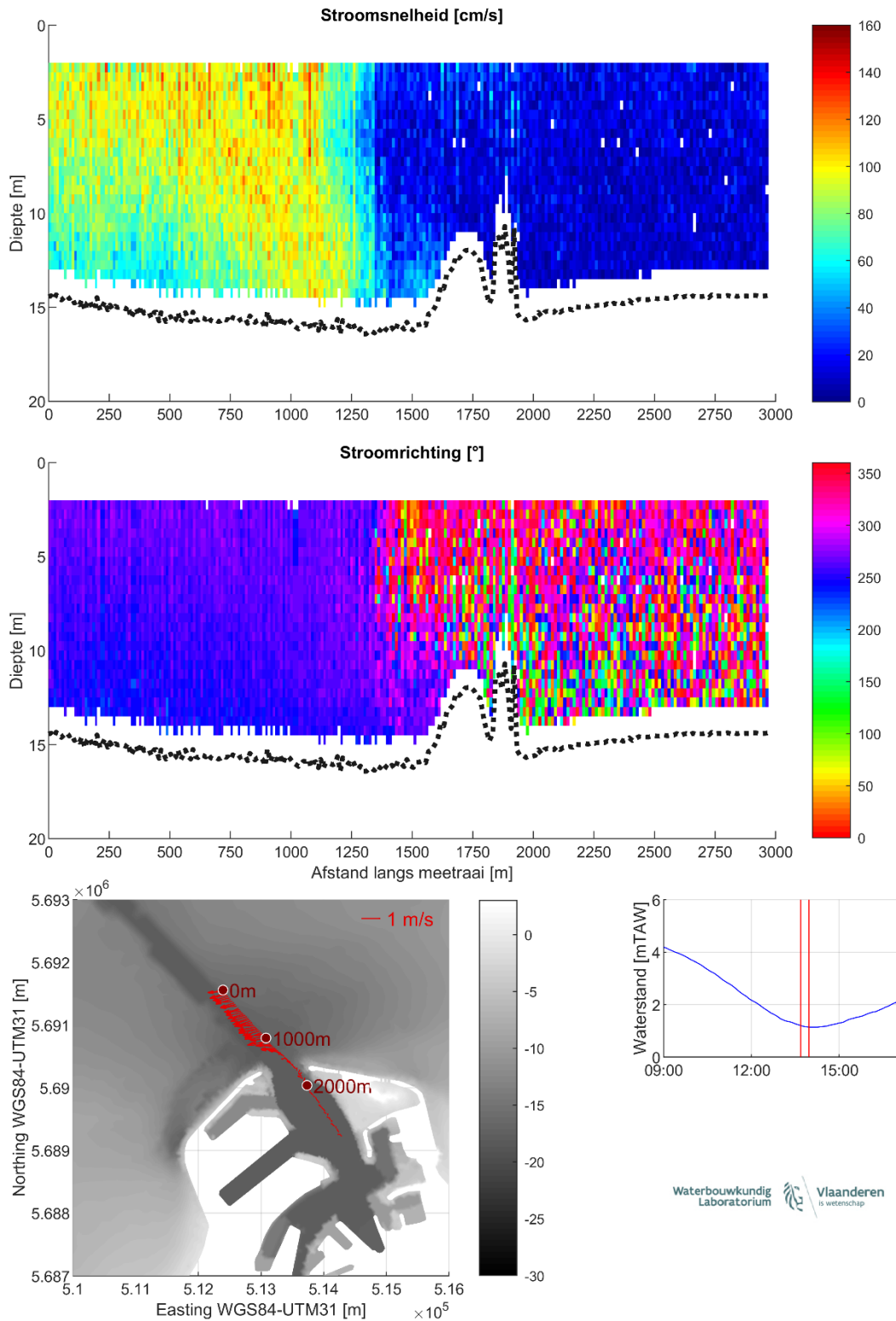
Figuur 21 – Stroomgegevens 09/08/2023 raai 16: snelheids grootte (top), -richting (midden) en diepte-gemiddelde vectoren (onder)
