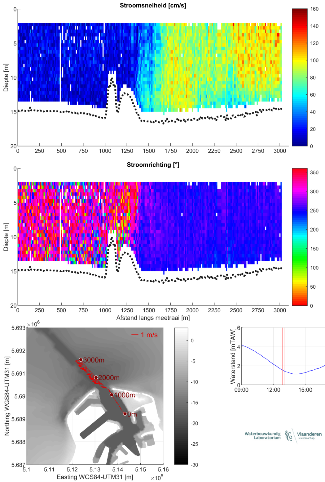
Figuur 18 – Stroomgegevens 09/08/2023 raai 13: snelheids grootte (top), -richting (midden) en diepte-gemiddelde vectoren (onder)
