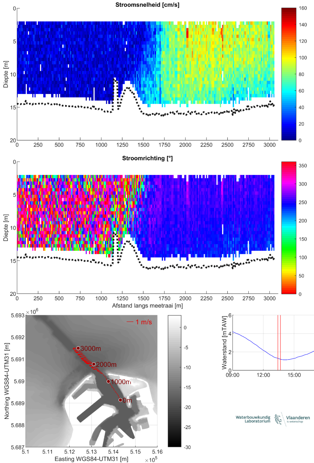
Figuur 20 – Stroomgegevens 09/08/2023 raai 15: snelheids grootte (top), -richting (midden) en diepte-gemiddelde vectoren (onder)
