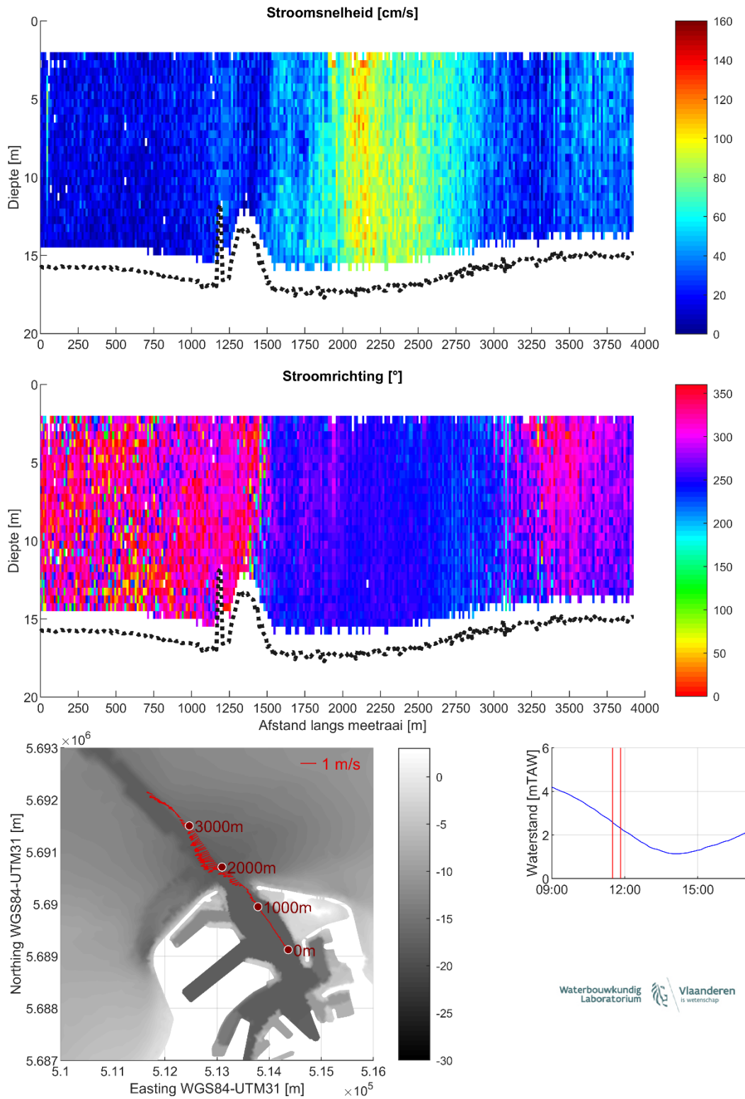
Figuur 14 – Stroomgegevens 09/08/2023 raai 9: snelheids grootte (top), -richting (midden) en diepte-gemiddelde vectoren (onder)
