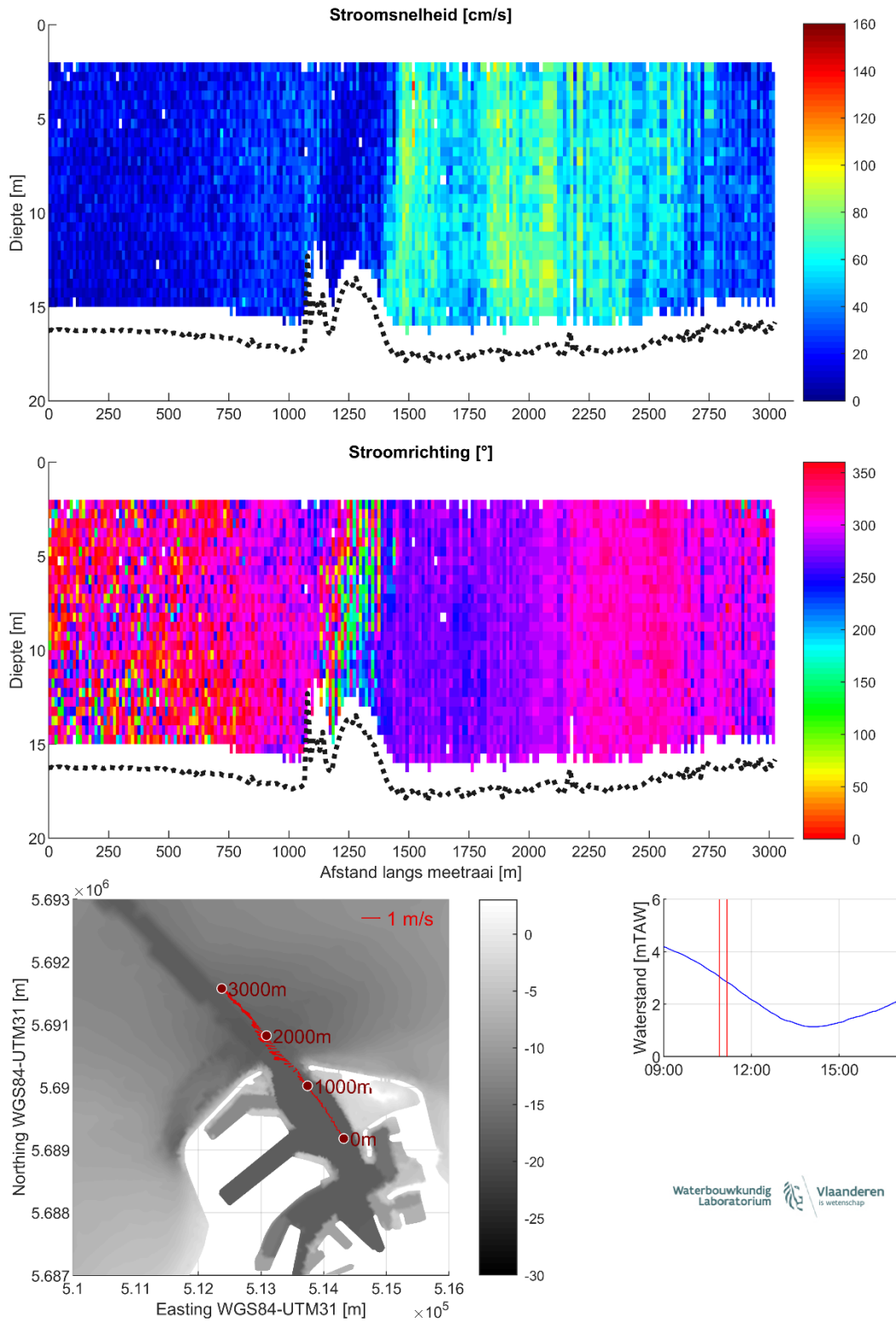
Figuur 12 – Stroomgegevens 09/08/2023 raai 7: snelheids grootte (top), -richting (midden) en diepte-gemiddelde vectoren (onder)
