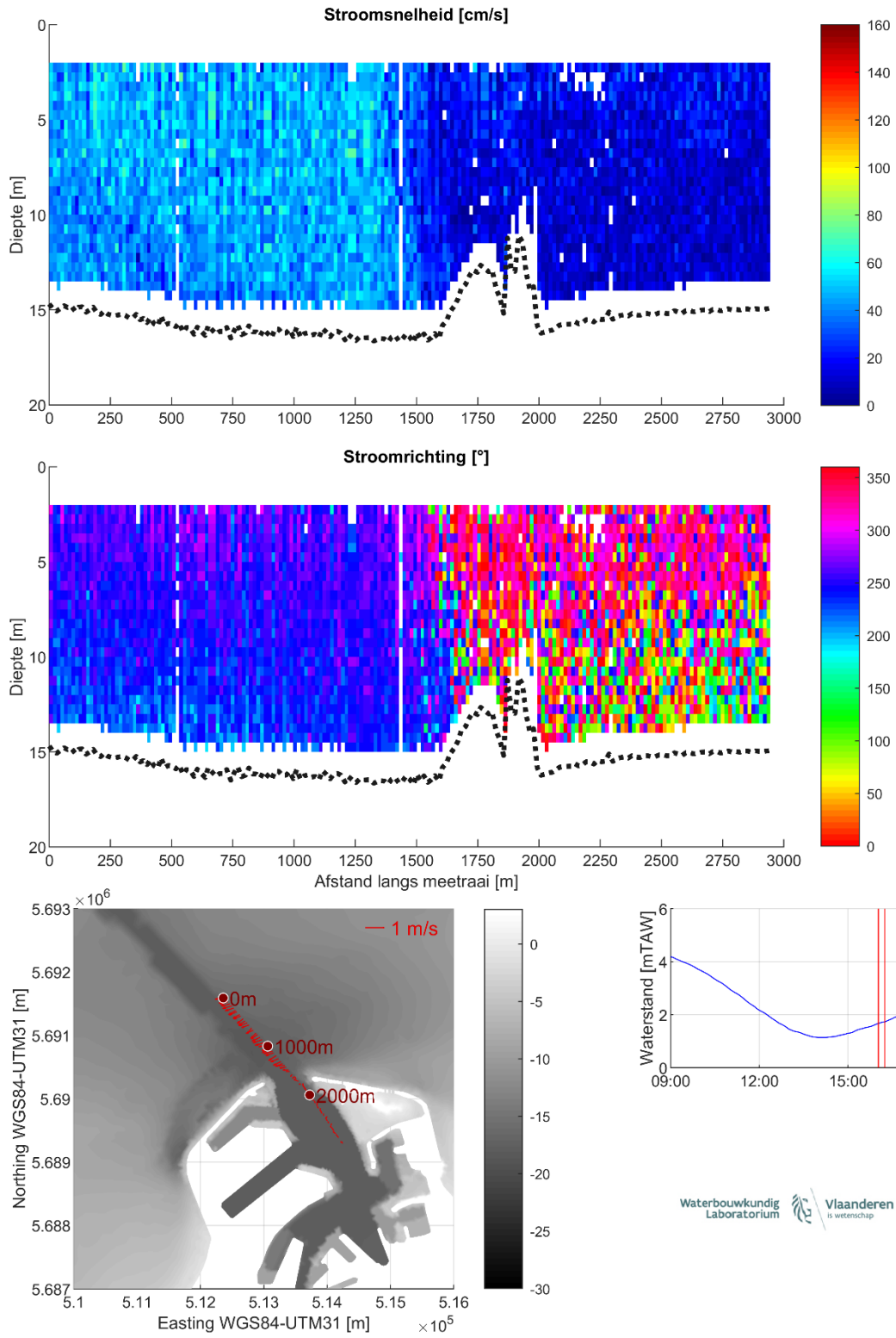
Figuur 29 – Stroomgegevens 09/08/2023 raai 24: snelheids grootte (top), -richting (midden) en diepte-gemiddelde vectoren (onder)
